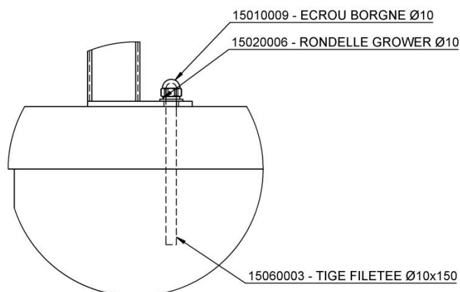
DÉTAIL A ECHELLE 1 : 5
