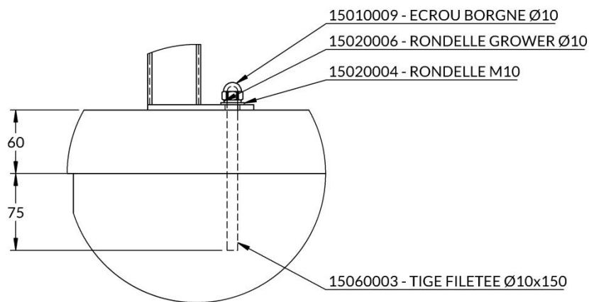
DÉTAIL A ECHELLE 1 : 5
