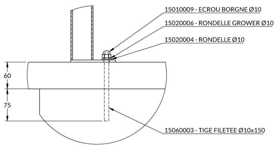
DÉTAIL B ECHELLE 1 : 5
