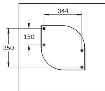
COUPE A-A ENTRAXE SCHELLEMENT
