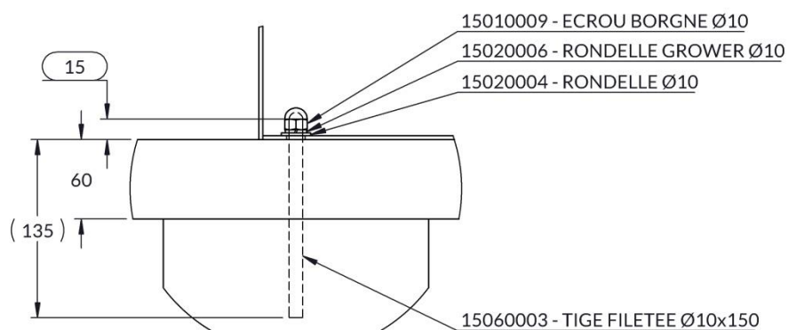
DÉTAIL B ECHELLE 1 : 5
