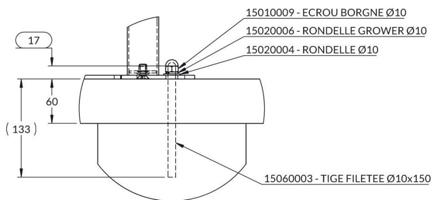
DÉTAIL B ECHELLE 1 : 5
