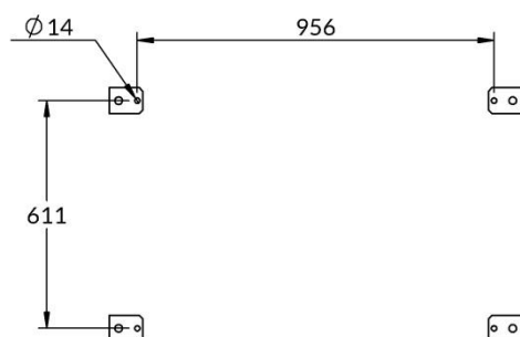
COUPE A-A
