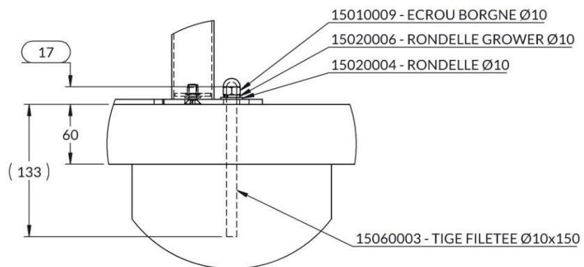
DÉTAIL B ECHELLE 1:5
